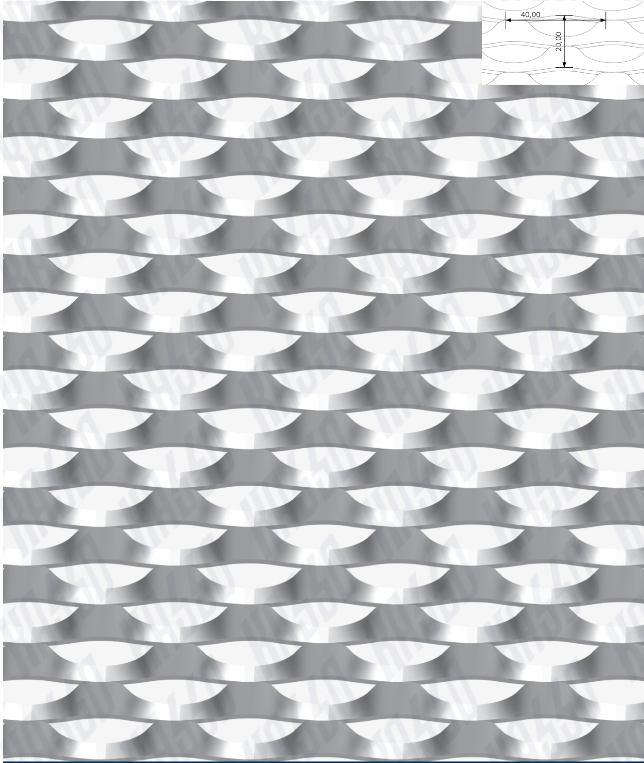
GM4020 / 40,00x20,00(22.00)x8,00x2,00mm - Geçirgenlik Oranı / Open Area Ratio (%): 33
