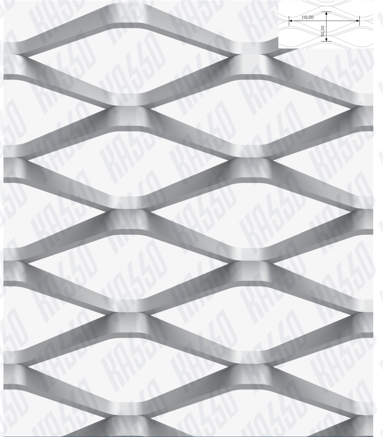
GM11550 / 115,00x50,00(48,00)x12,00x3,00mm - Geçirgenlik Oranı / Open Area Ratio (%): 50
