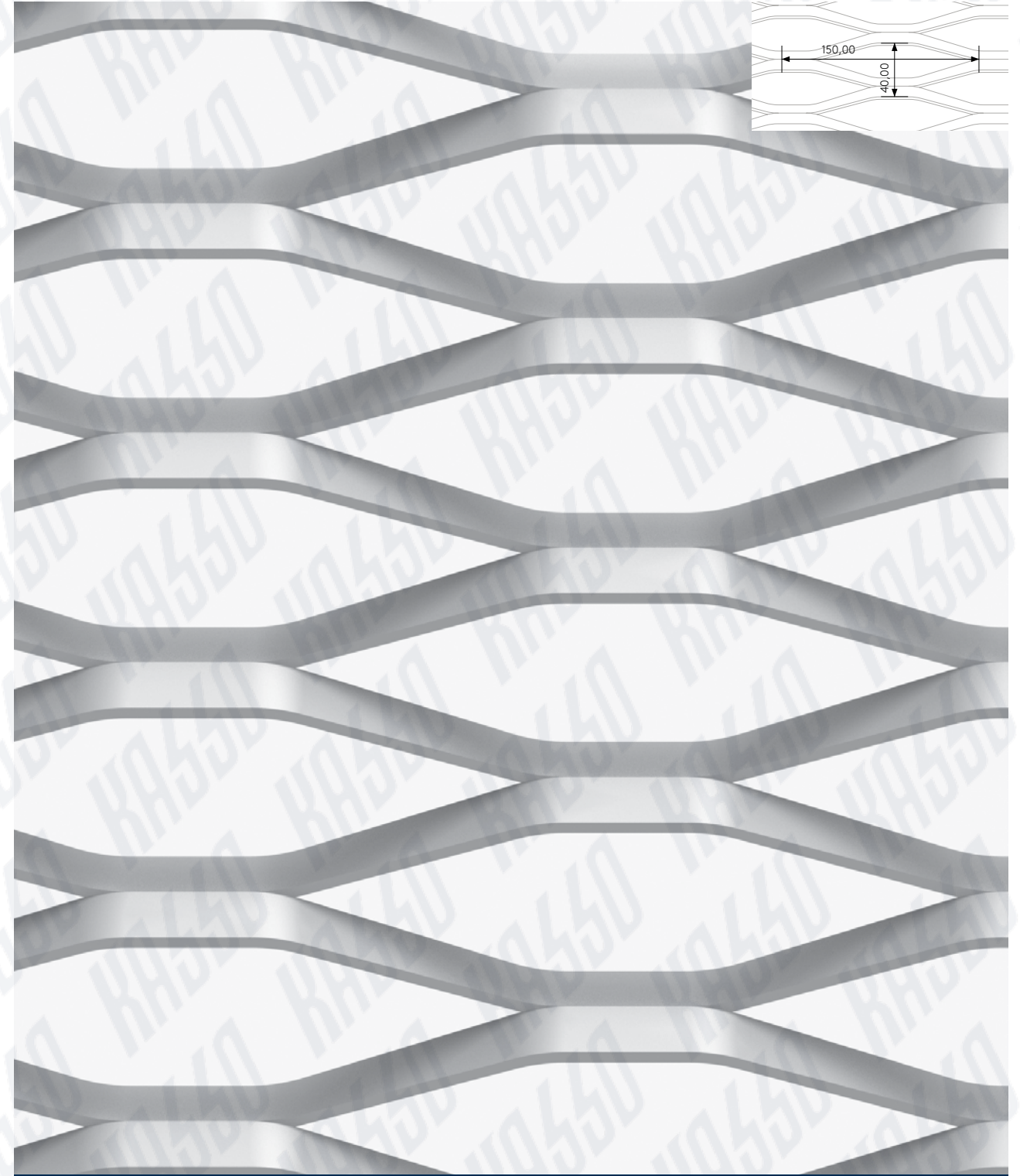
GM15040 /150,00x40,00(44.00)x9,40x2,00mm - Geçirgenlik Oranı /Open Area Ratio (%) : 52 Ölçek /Scale 1:1
